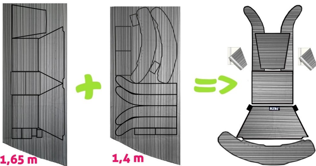
Celošátkové nosítko + (2x) jednostranné slintáčky – horizontální stříh, sesazený
