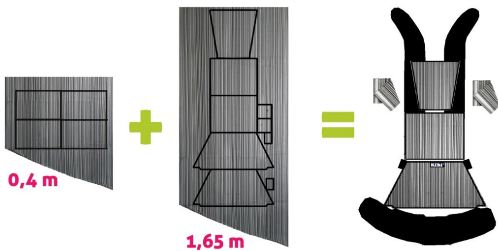
Kombinované nosítko + oboustranné slintáčky (nebo 2x jednostranné) – vertikální střih, sesazený
